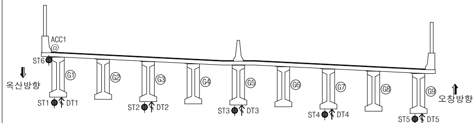
A-A단면 부착위치
