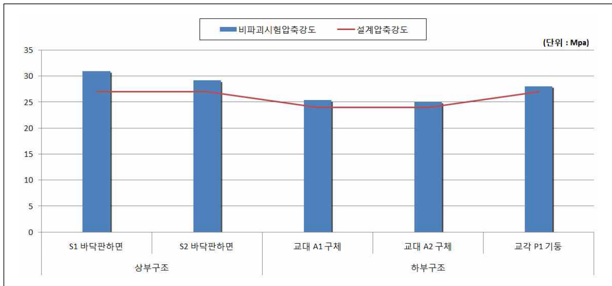
【그림 2.11.6】 콘크리트 강도시험 결과 그래프
